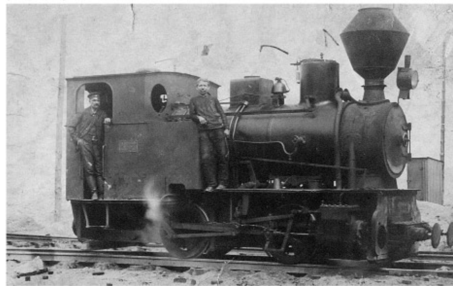
Parowóz kolei wąskotorowej, ok. 1912 r.
