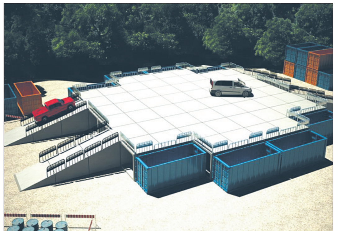
Wizualizacja przykładowej rampy rozładunkowej w Punkcie Selektywnej Zbiórki Odpadów Komunalnych
