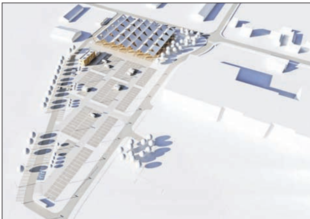
Układ przestrzenny planowanego targowiska
