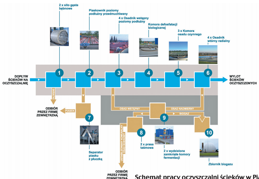
Schemat pracy oczyszczalni ścieków w Piasecznie
